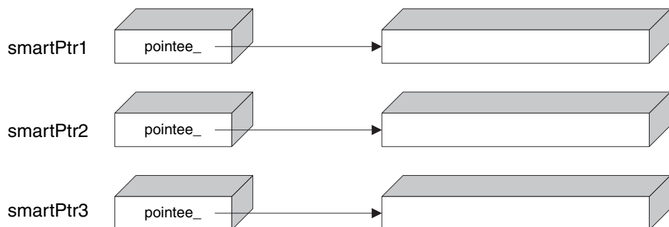
图 7.1: 具有深度复制的智能指针的内存布局
